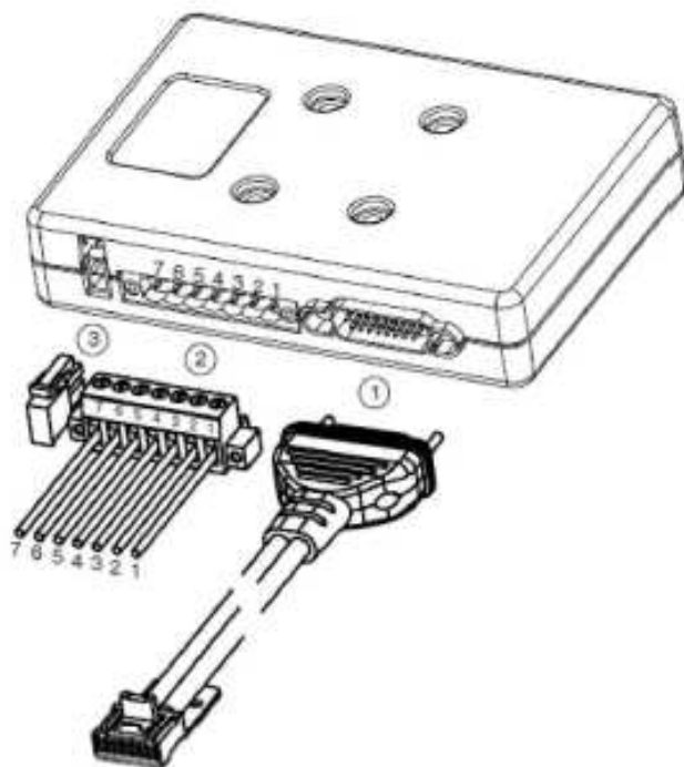
Figura 5. Fronte della junction box
