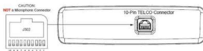
Figura 3. Retro del frontellino remoto
