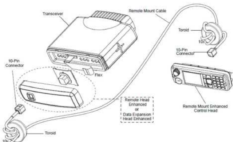
Figura 1. Corpo centrale e frontellino remoto
